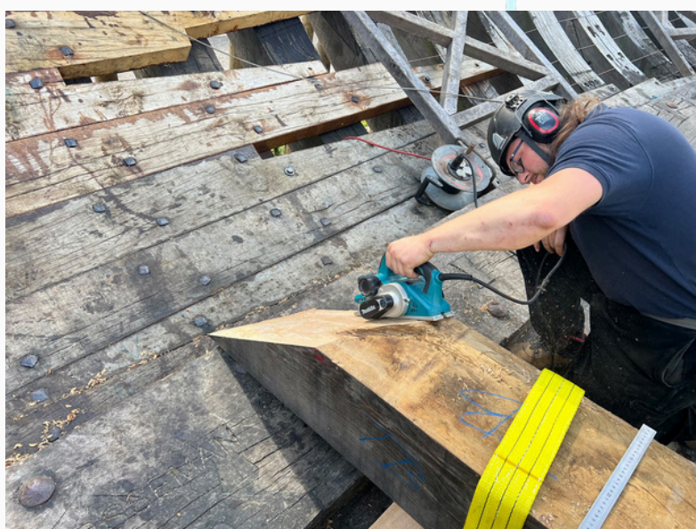
Ajustage des coupes de bout du barrot
